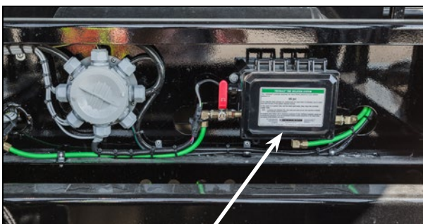
Figure 20 – Boîtier de commande de gonflage des pneus
