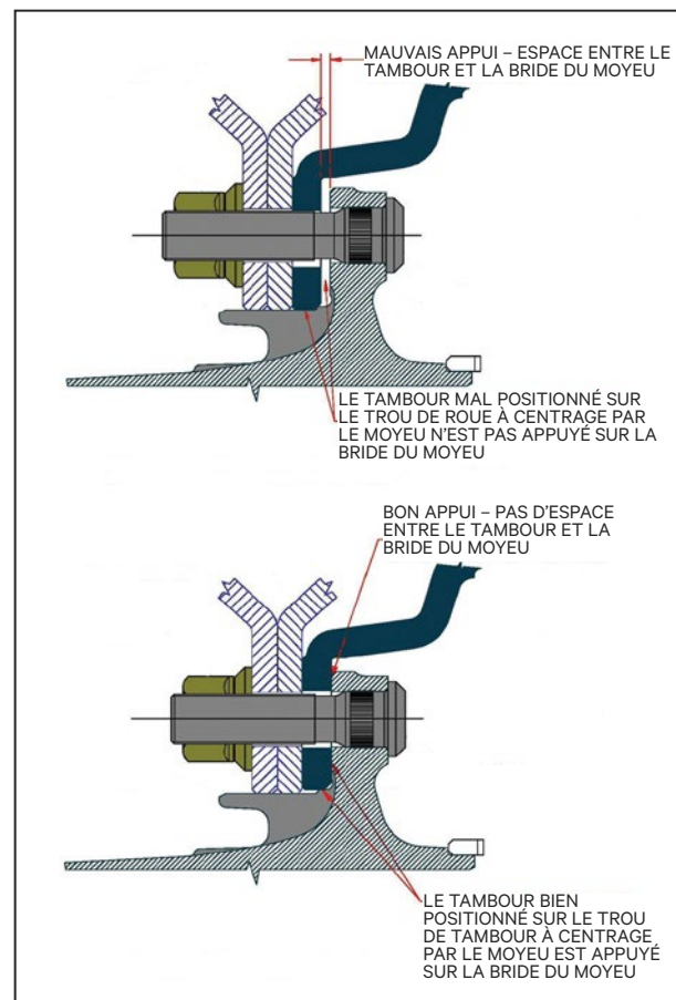
Figure 42 – Tambour de frein bien appuyé
