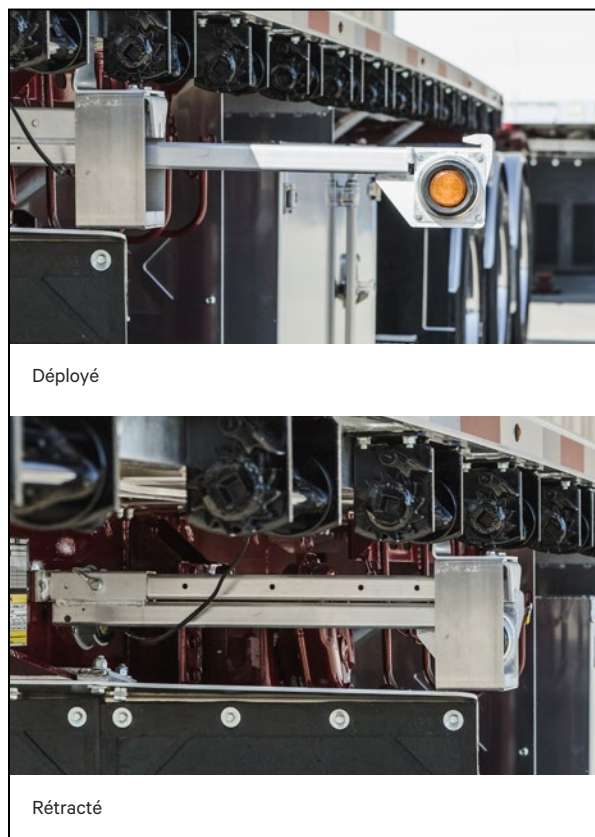
Figure 18 – Feux de gabarit en option
