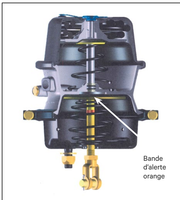
Figure 38 – Récepteur de frein
