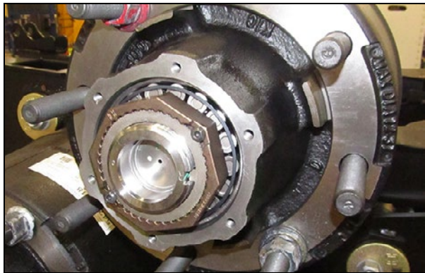
Figure 35A – Écrou Precision
