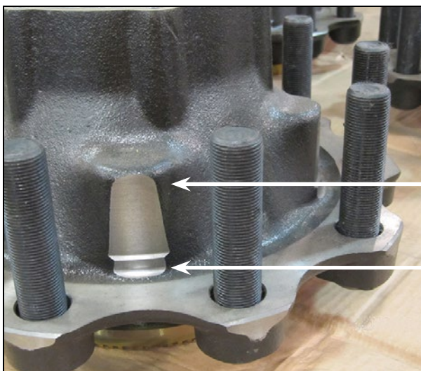
Figure 43 – Trous de centrage par le moyeu
