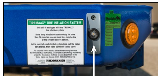
Figure 21 – Témoin de défektivité
